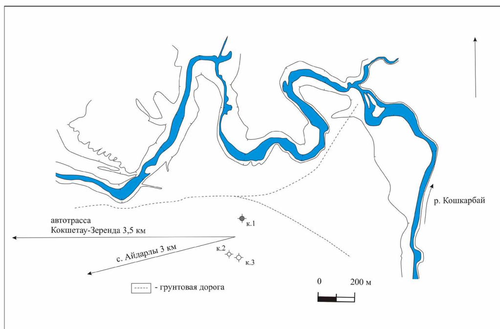
Рис. 1. Могильник Айдарлы. Топоплан
